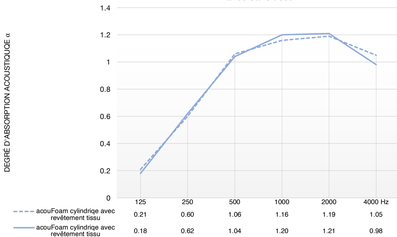
Degré d'absorption acoustique acouFoam absorbeur cylindrique avec/sans tissu
